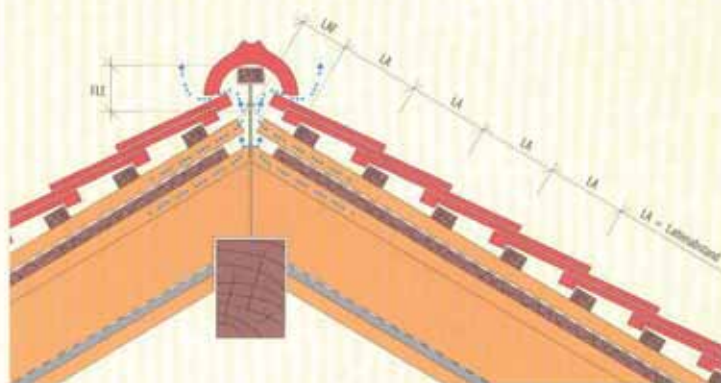
Provedení hřebene jednoduché krytí
