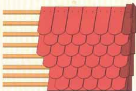
1) použití krajní bobrovky typ 3
