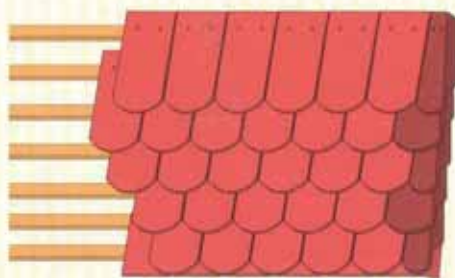
2) použití krajní bobrovky typ 6
