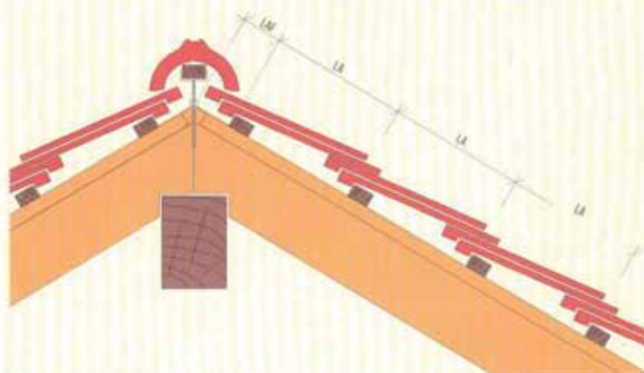
Provedení hřebene dvojité krytí
